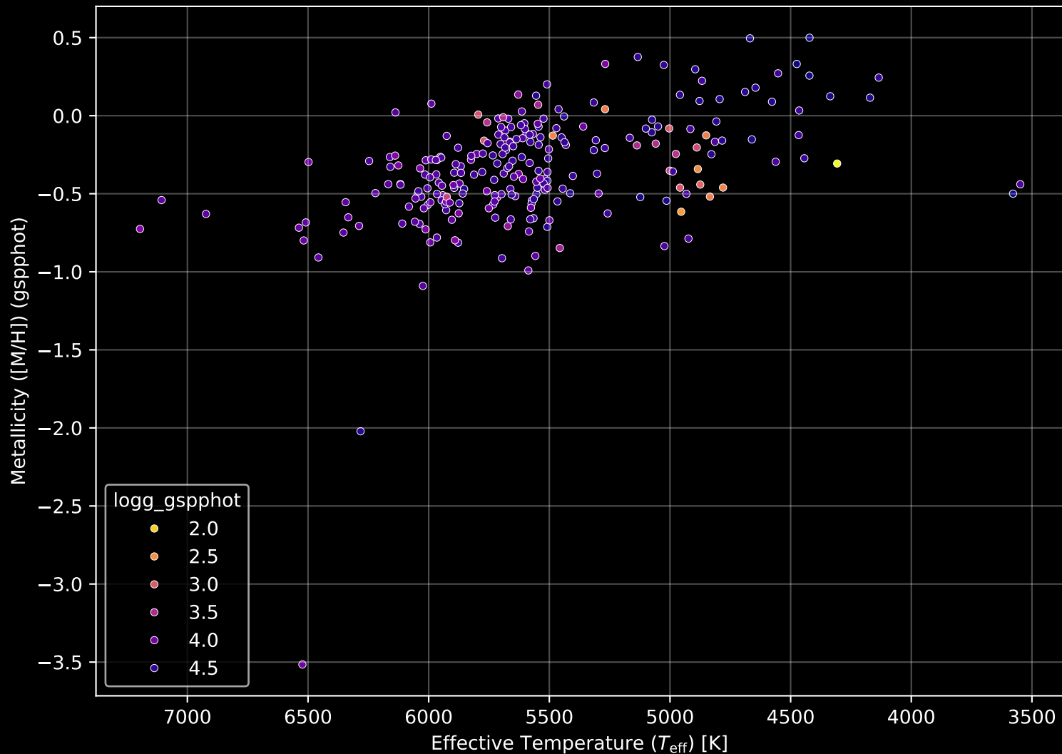
GALAH DR4 Field: [7032] Stellar Population Parameters (n= 248)
